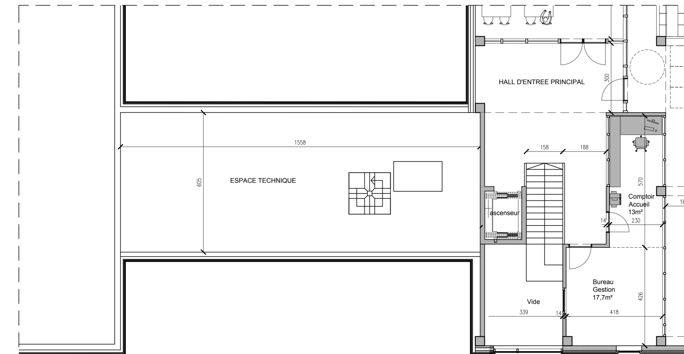
PLAN ETAGE TECHNIQUE - ECH.: 1/100
