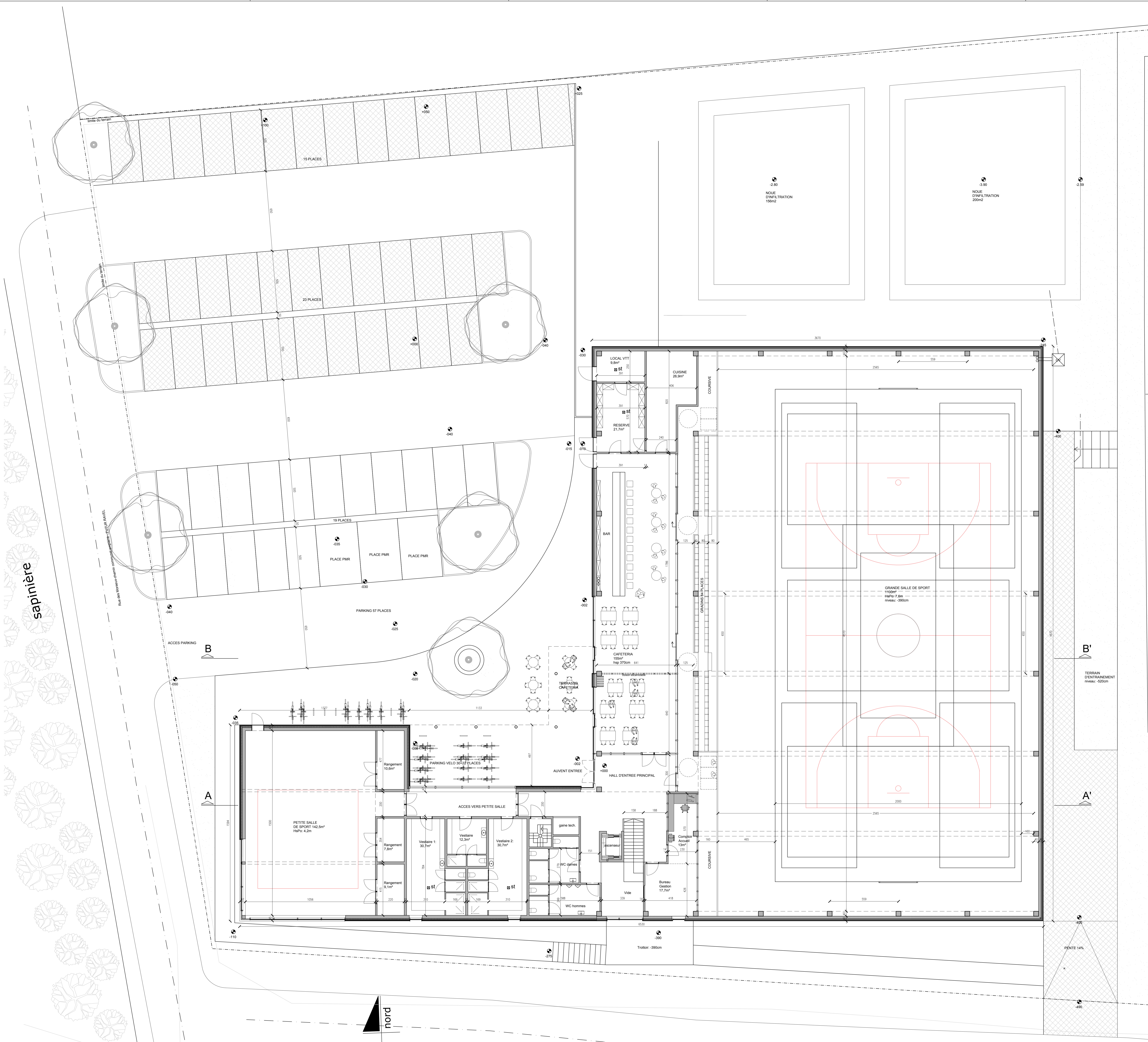
PLAN ETAGE = NIVEAU CAFETERIA ET PARKING - ECH.: 1/100
