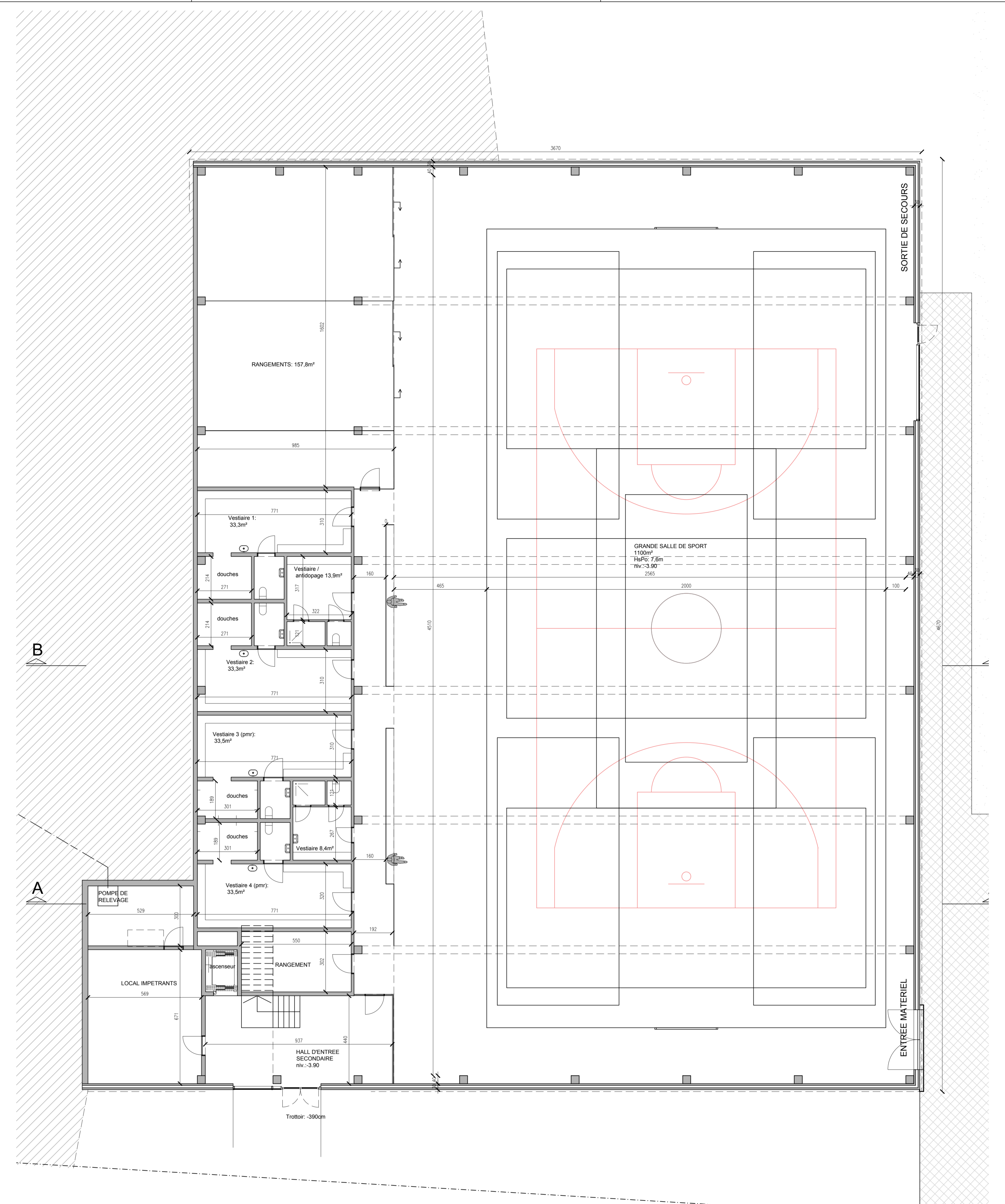
PLAN REZ = NIVEAU SALLE ET TERRAIN FOOT - ECH.: 1/100
